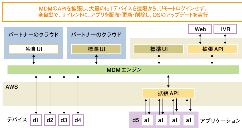
図 「BizMobile Go!」の IoT 管理概念図
